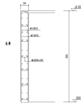
钢板布置做法大样1
