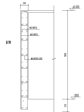
钢板布置做法大样2
